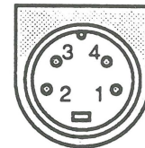
Mini DIN-4
