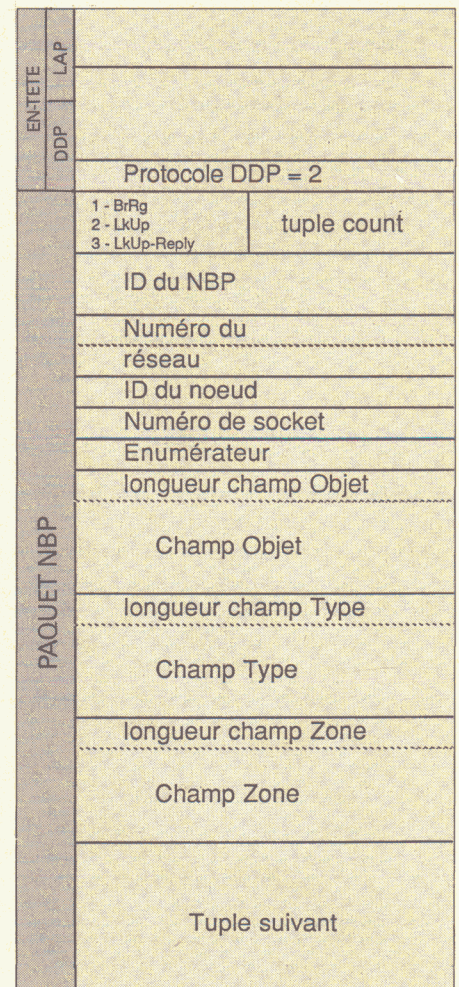
Figure 3 : paquet au format NBP.
