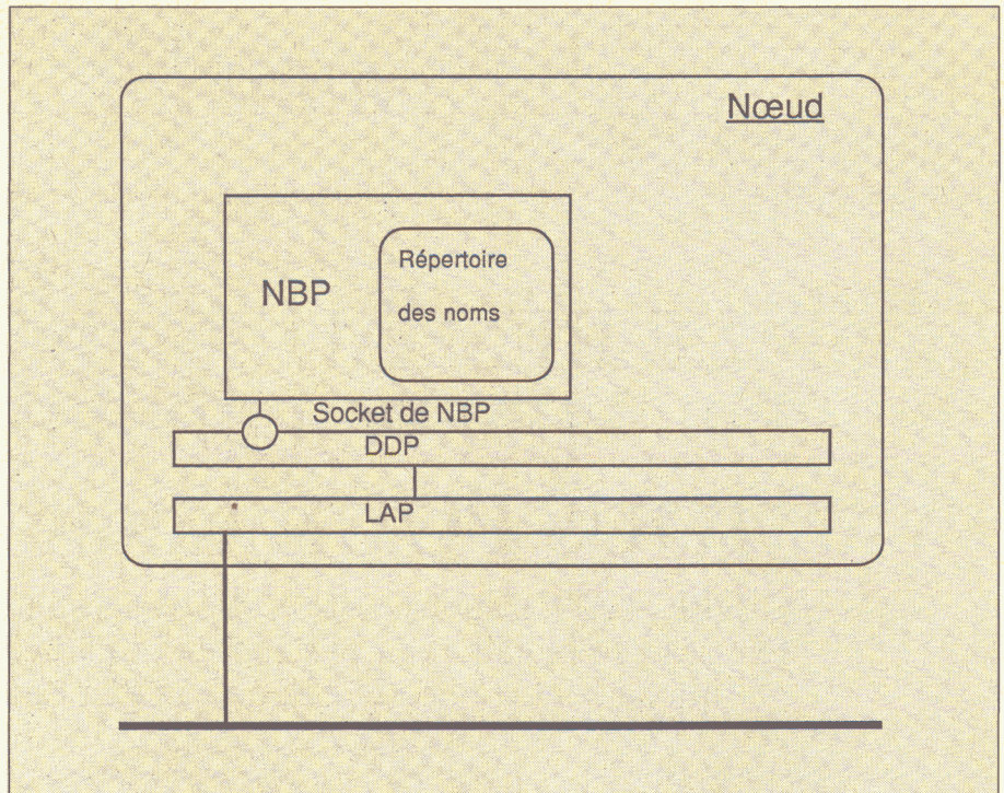
Figure 2 : répertoire des noms sur NBP, contenu dans chaque Macintosh et contenant les correspondances <Nom, Adresse de la prise (socket)>. (NBP : Name Binding Protocol)
