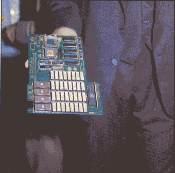
La carte de Levco, une vraie bombe électronique.
